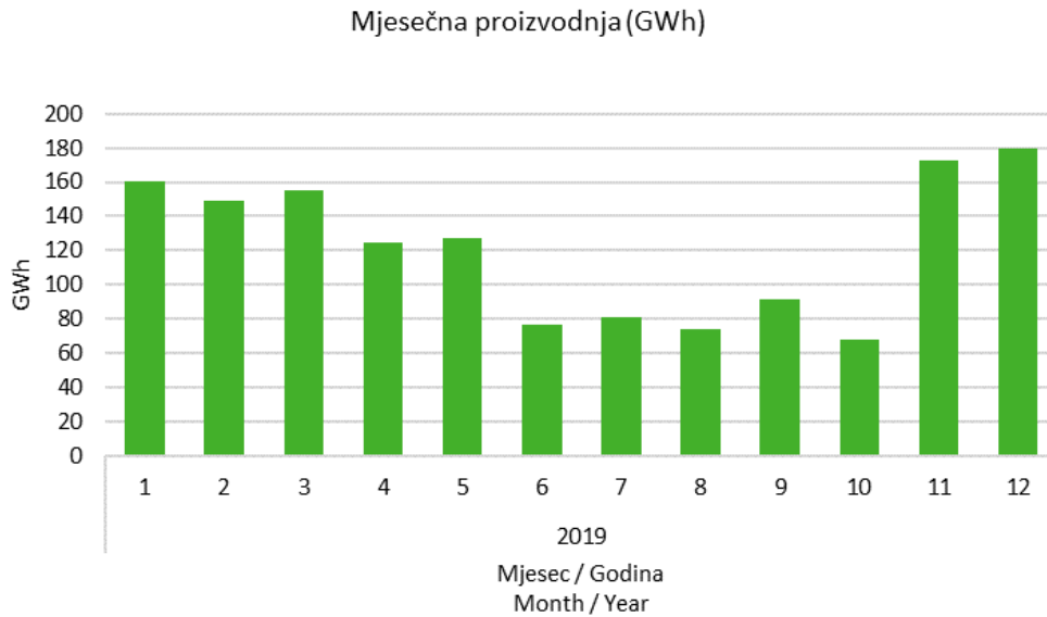
Slika 9 Mjesečna proizvodnja svih vjetroelektrana
