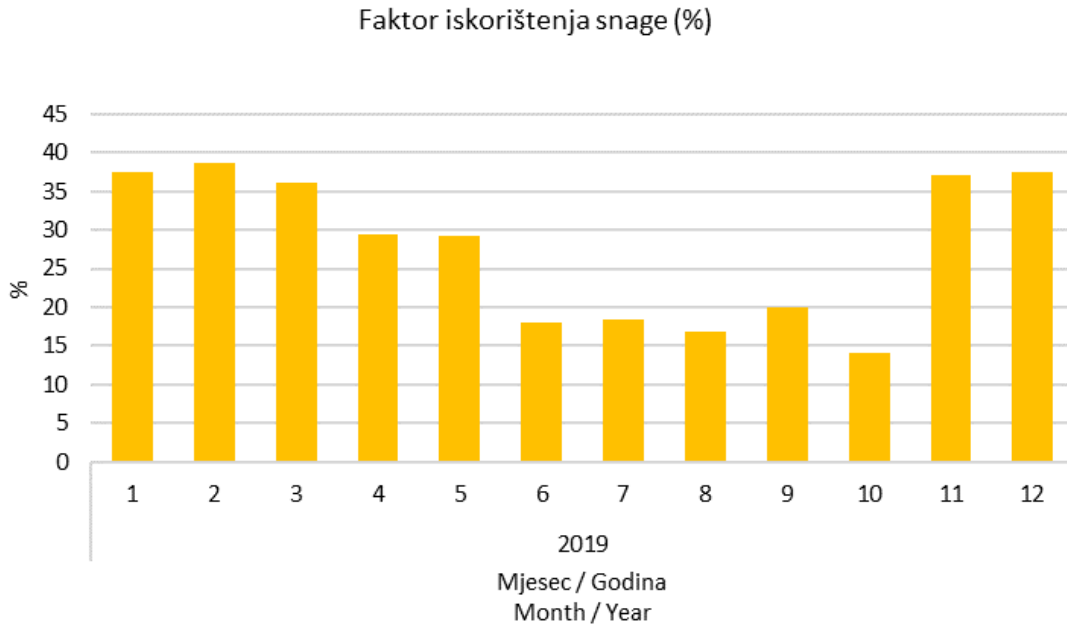
Slika 10 Mjesečni faktor iskorištenja snage svih vjetroelektrana
